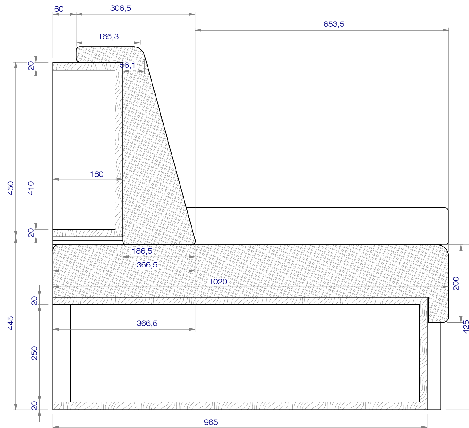
SEZ. C-C
