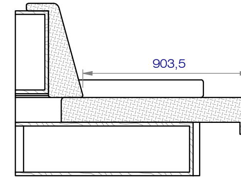
SEZ. D-D
